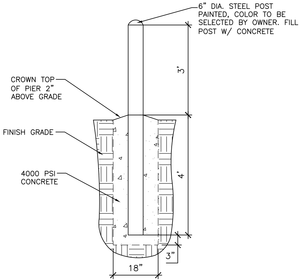
BOLLARD DETAIL SCALE: 1/2" = 1'-0"
